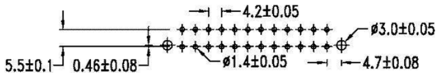
P.C.B. hole dimensions
