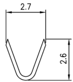
A-A SECTION
