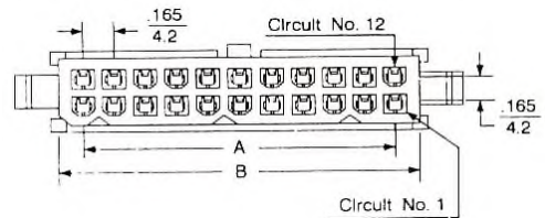
22 Circuits
