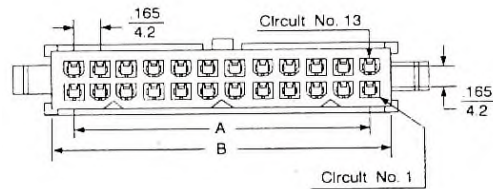
24 Circuits
