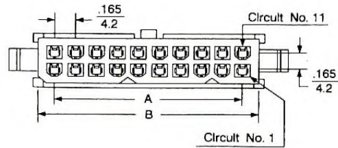
20 Circuits
