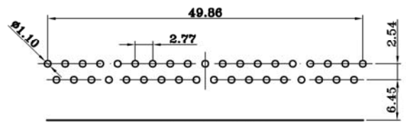
PCB LAYUOT
