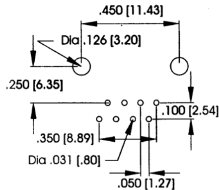
8P8C
