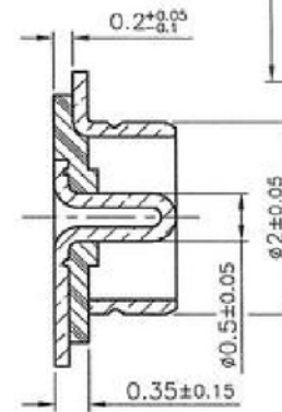
A-A' SECTION (A-A' 剖面)
