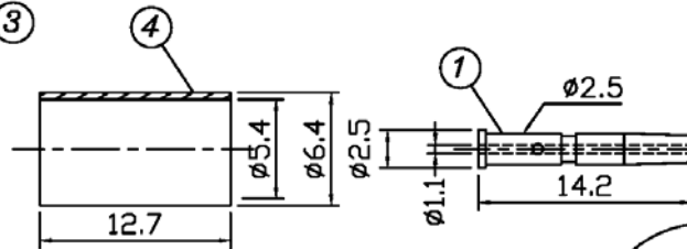
FERRULE
