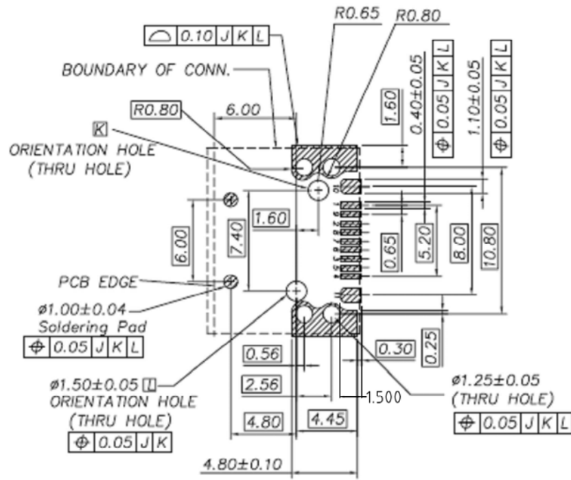
PCB LAYER OUT SCALE 5:1
