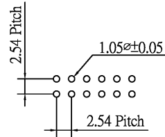
P.C.Board Layout
