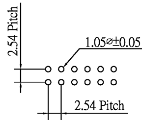
P.C.Board Layout
