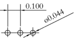
P.C.Board Layout
