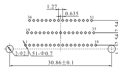
DSM51-FT-E-J
