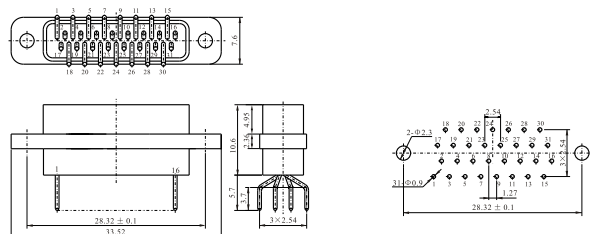
DSM31-FT-R
