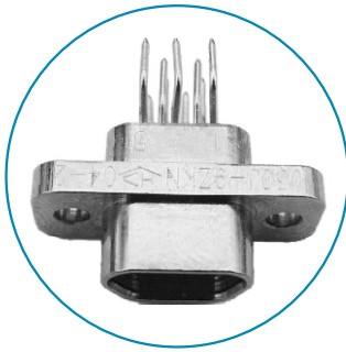
DSM09-FT-R
