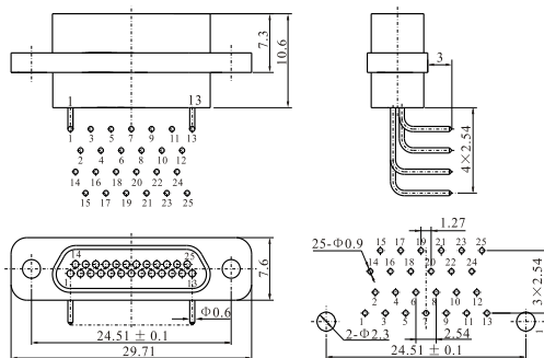
DSM25-FT-E
