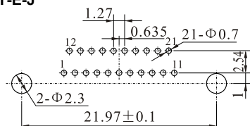
DSM21-FT-E-J
