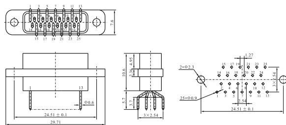
DSM25-FT-R
