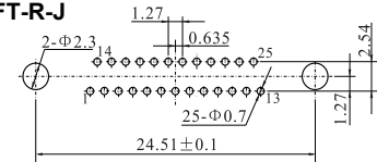
DSM25-FT-R-J
