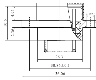
DSM51-FT-S
