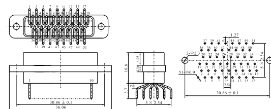
DSM51-FT-R
