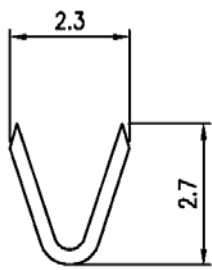
A-A SECTION
