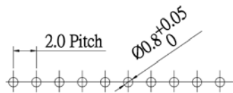
P.C.Board Layout
