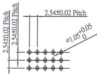
P.C.Board Layout
